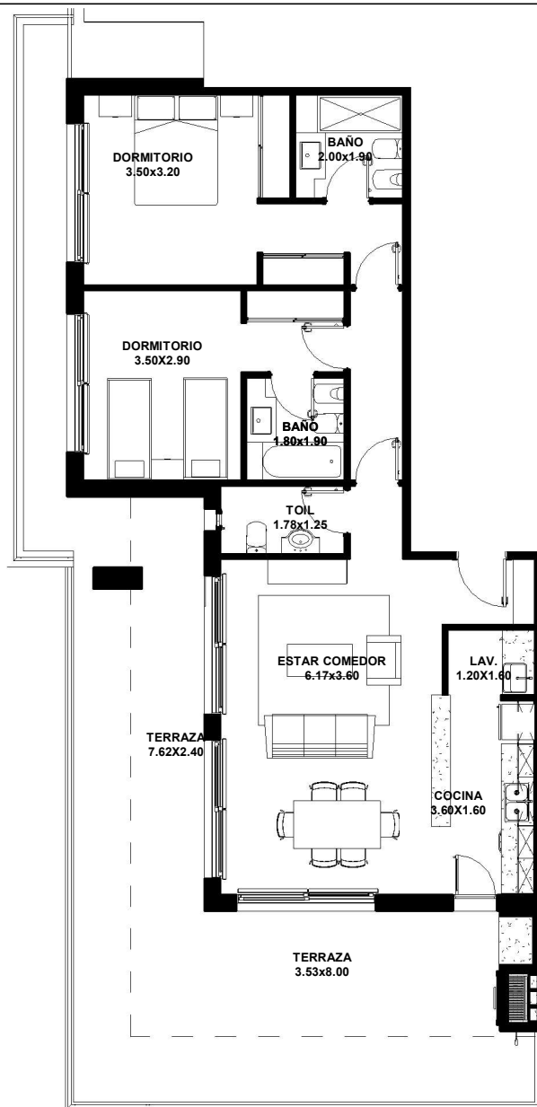
2 EDIFICIO 2 - U 301 1 : 125
