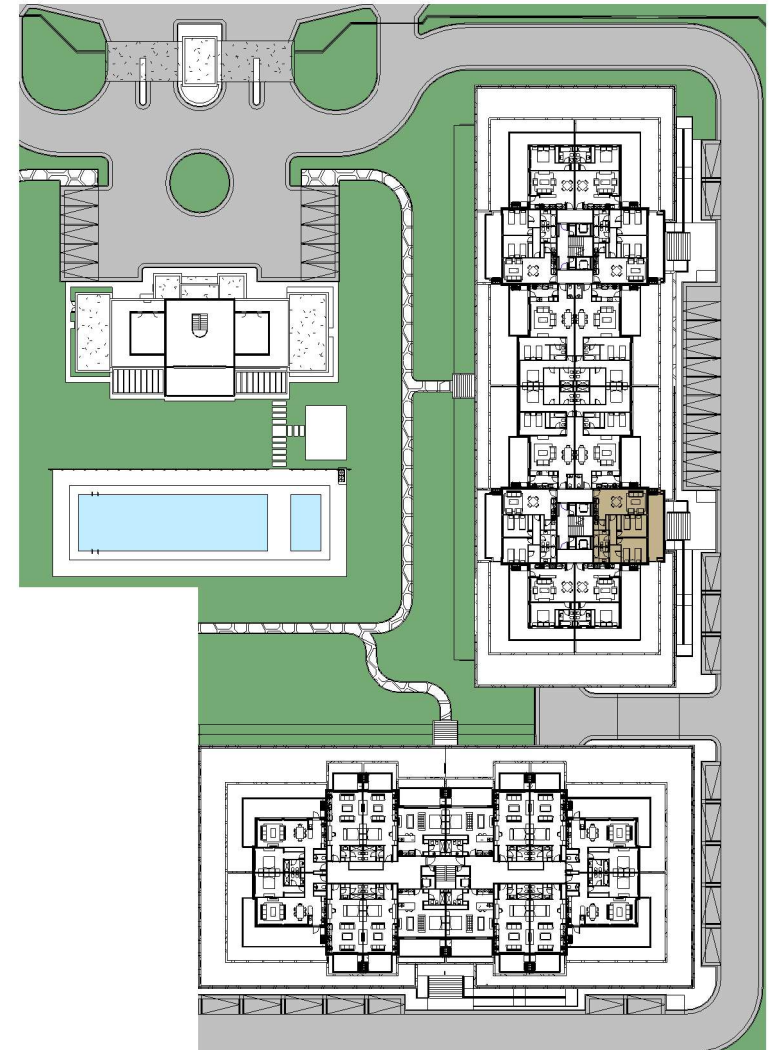
1 UBICACION 1 : 1000
